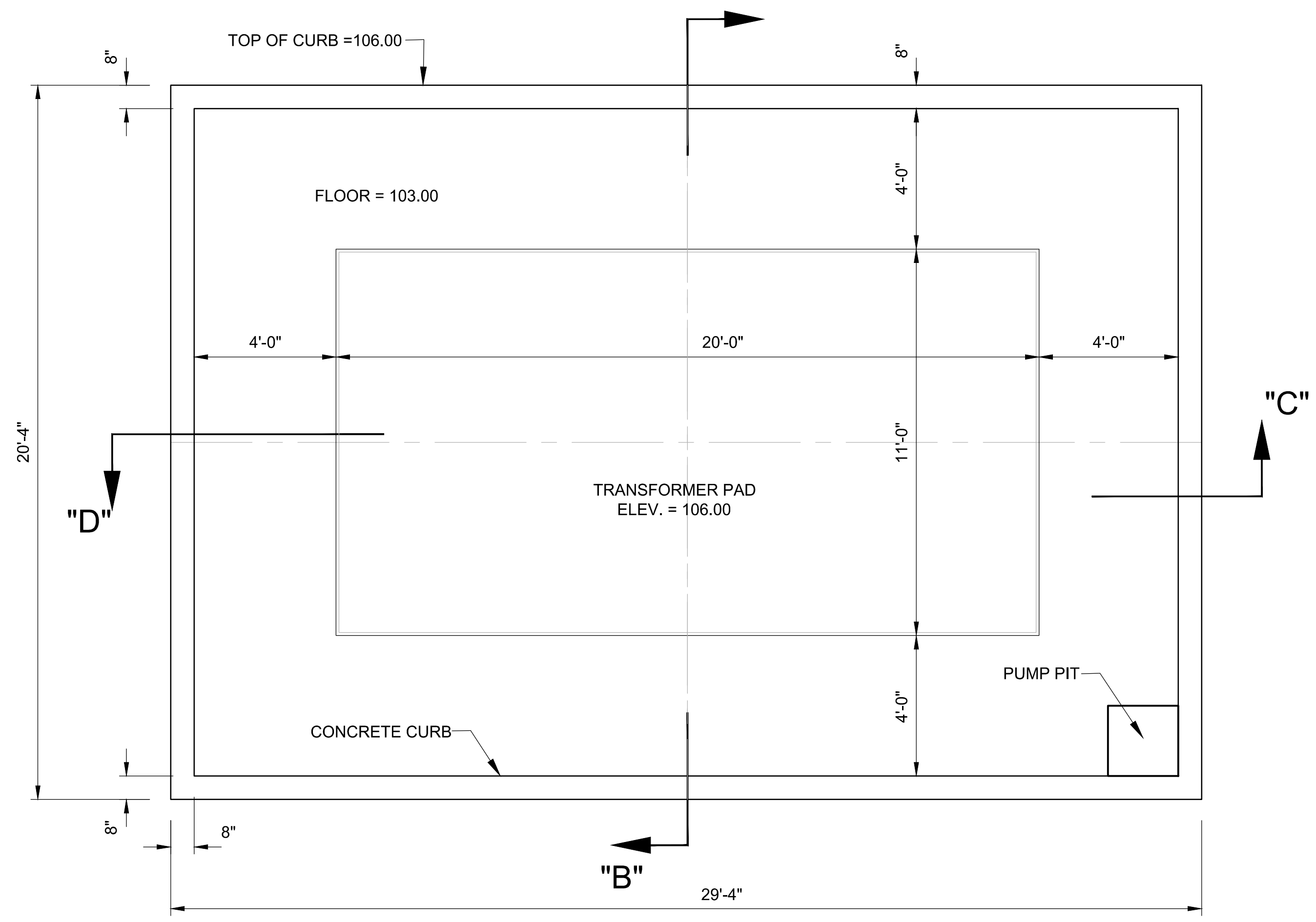
PLAN VIEW N.T.S.
