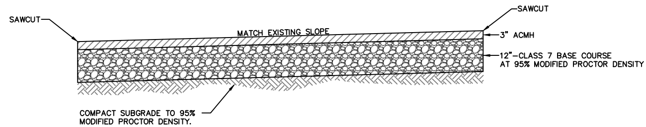
REPAIR TYPE 2 DETAIL N.T.S.
