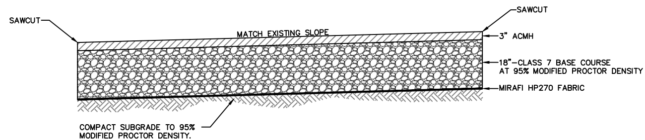
REPAIR TYPE 3 DETAIL N.T.S.
