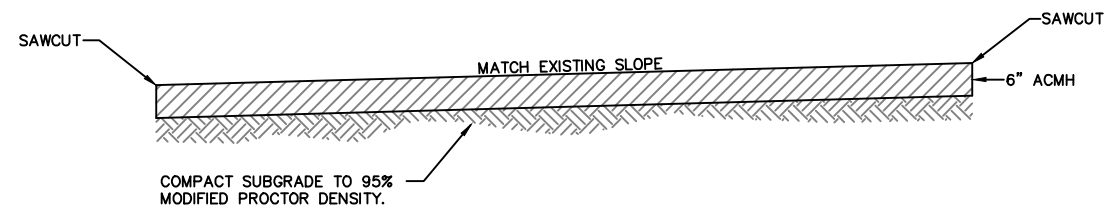
REPAIR TYPE 1 DETAIL N.T.S.
